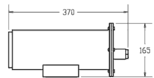
YHT400B Side view
