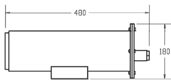
YHT400A Side view
